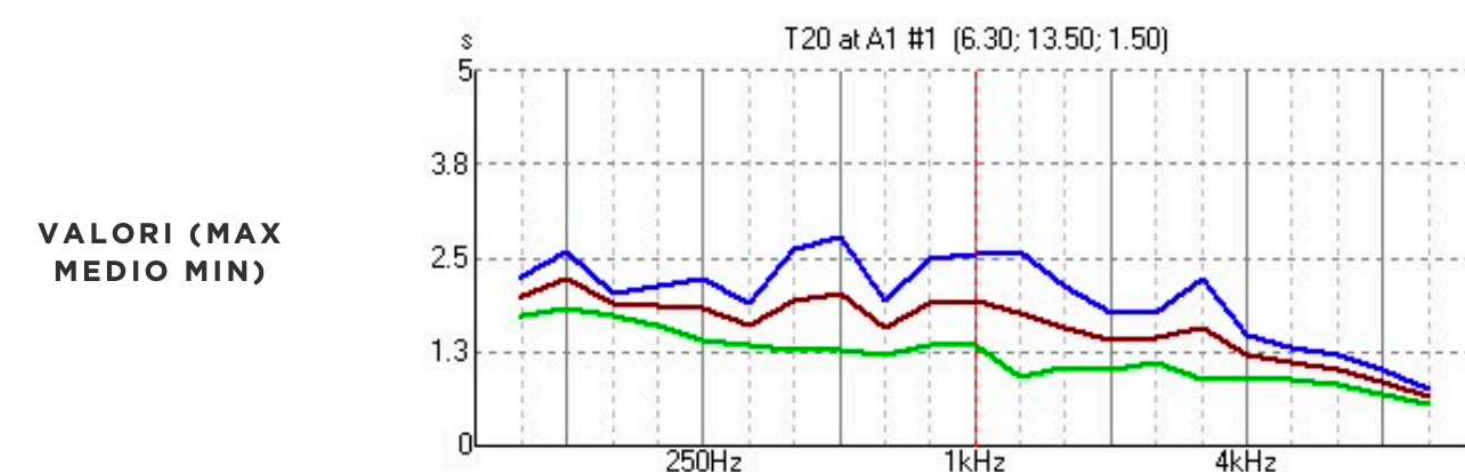
T20 - TEMPO DI RIVERBERAZIONE
