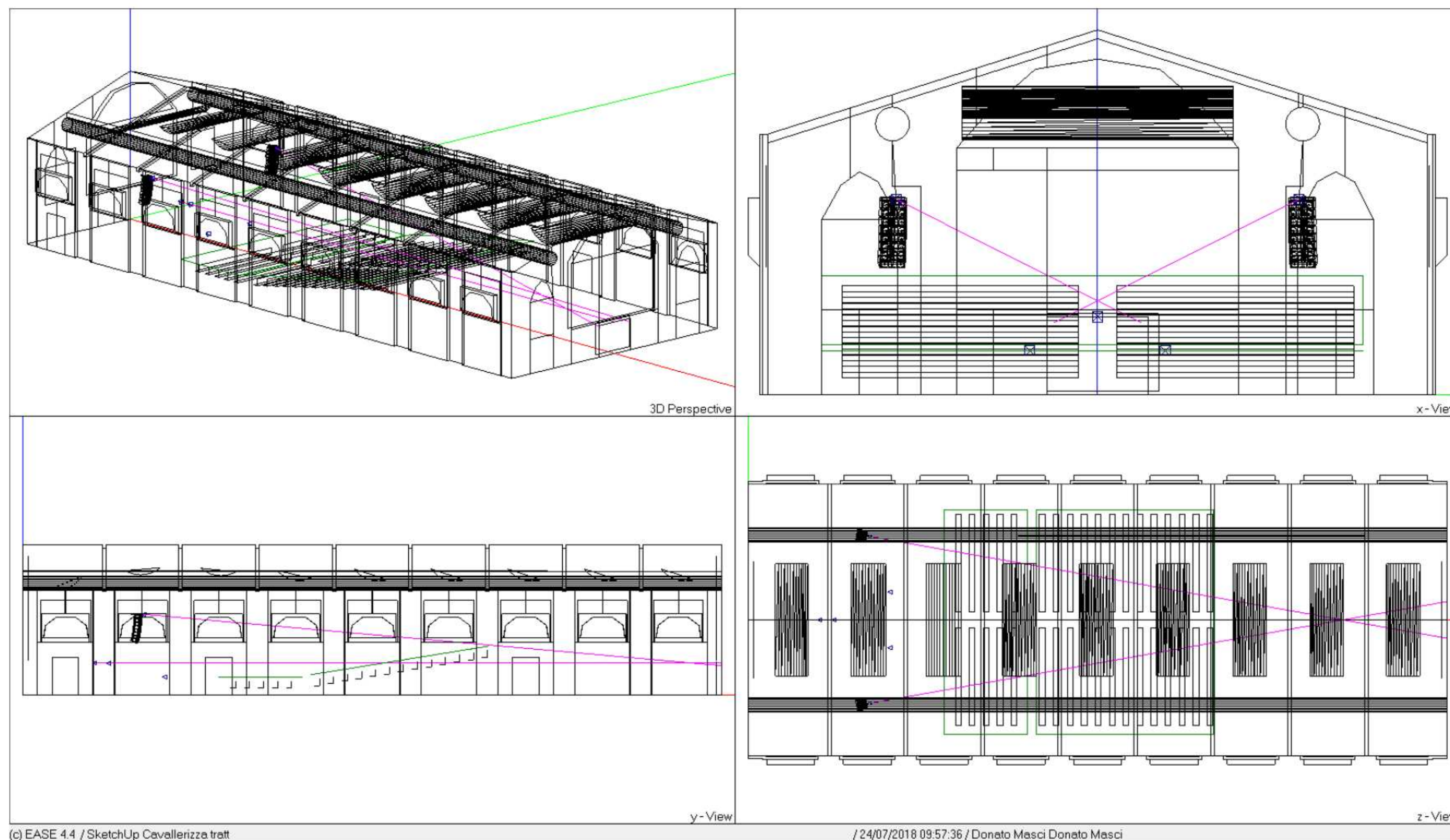
Modello 3d per studio al cad acustico
