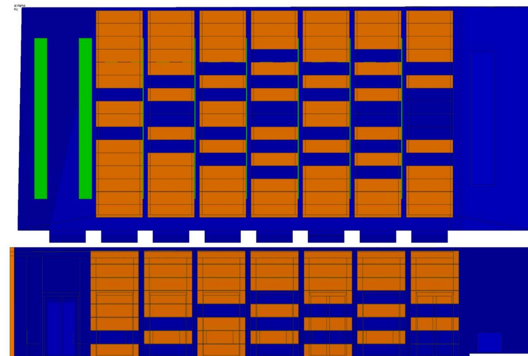
Disposizione pannelli lisci (in blu) e forati (in arancione) in pianta (sopra) e in sezione (sotto)
