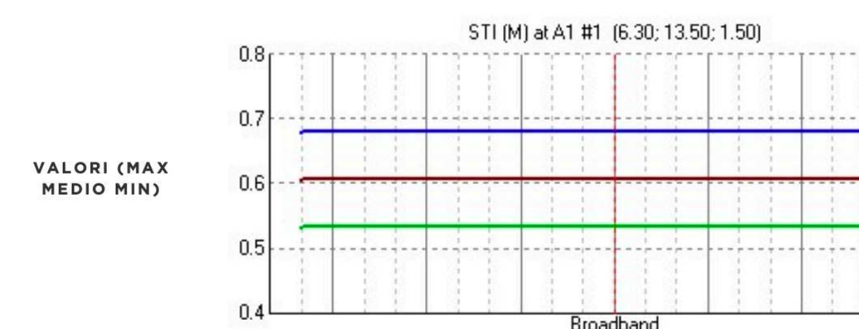
STI - INTELLIGIBILITÀ DEL PARLATO
