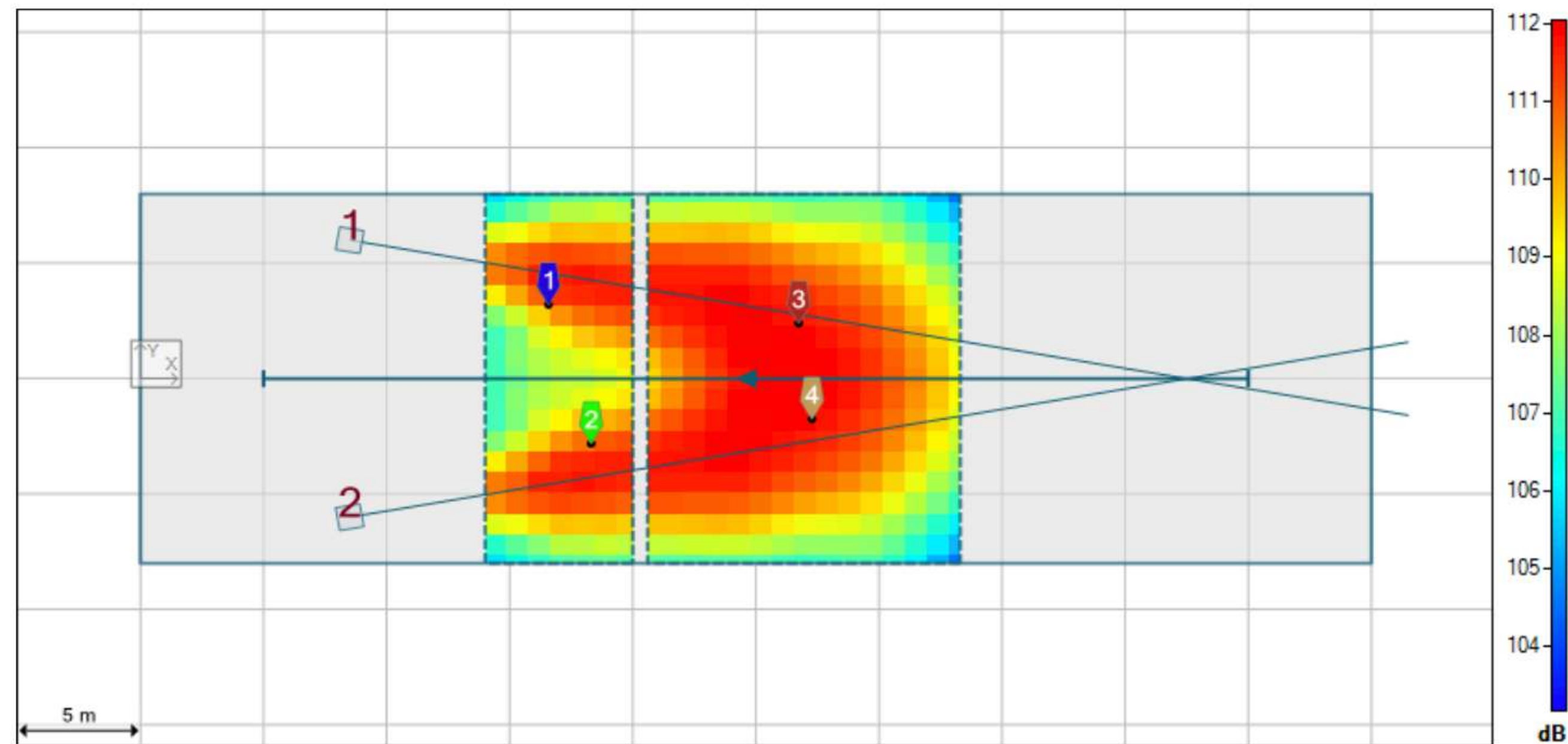
Copertura SPL diretta in pianta
