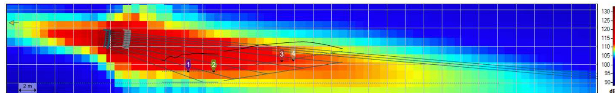
Copertura SPL diretta in sezione
