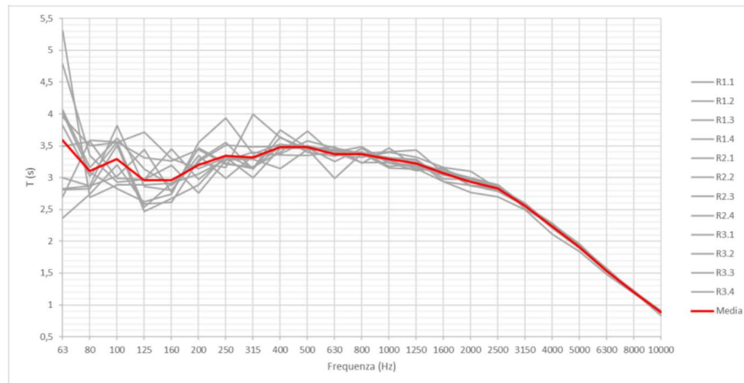
Tempi di riverberazione ( T_{30} ) misurati ante operam
